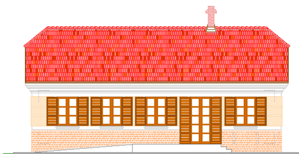
déli homlokzati vázlat
